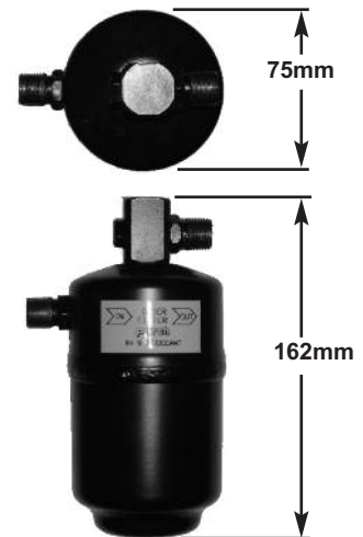
No6 MIO x No6 MIO PART No: 2700-10015
