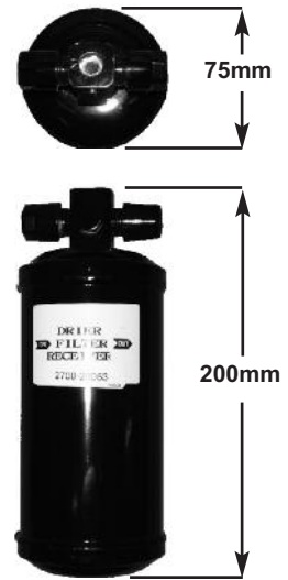
No6 MIO x No6 MIO 2 x 3/8" UNF PORTS PART No: 2700-20053
