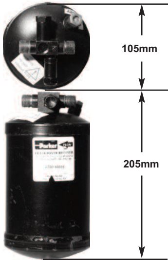
No6 MIO x No6 MIO RELIEF VALVE 1 X 3/8" UNF PORT PART No: 2700-10005
