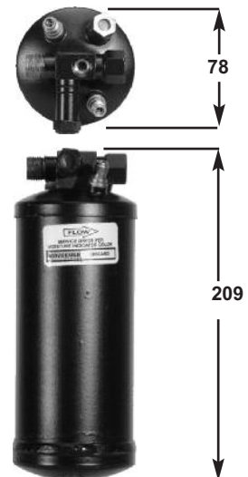
No6 MIO x No6 FIO 2 x 10mm MALE SWITCH PORT 1 x RELIEF VALVE
