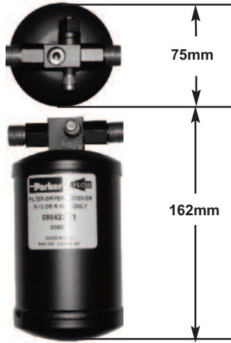
No6 MIO x No6 MIO 1 X 7/16" UNF PORT FUSE PLUG PART No: 2700-10006
