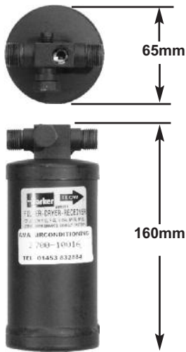
No6 MIO x No6 MIO PART No: 2700-10016
