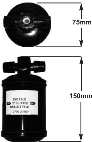
No6 MIO x No6 MIO 2 x 3/8" UNF PORTS PART No: 2700-20050
